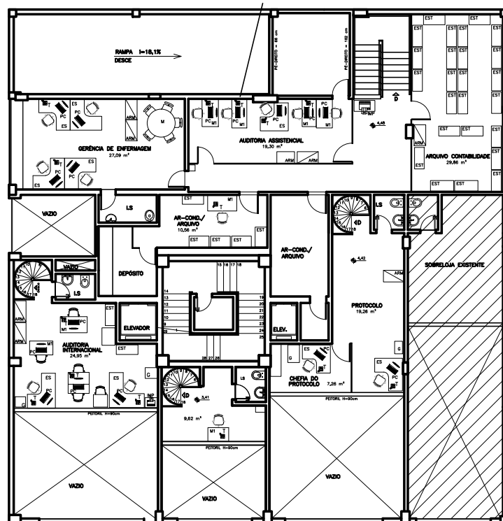
PLANTA SOBRELOJAS ESCALA 1:125 ÁREA TOTAL OCUPADA: 278,80m 2
